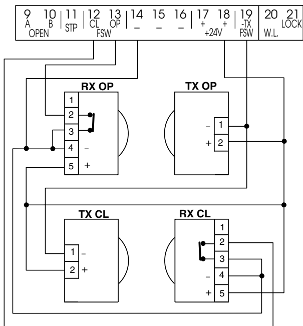
Conexión de una pareja de fotocélulas en apertura y otra en cierre
